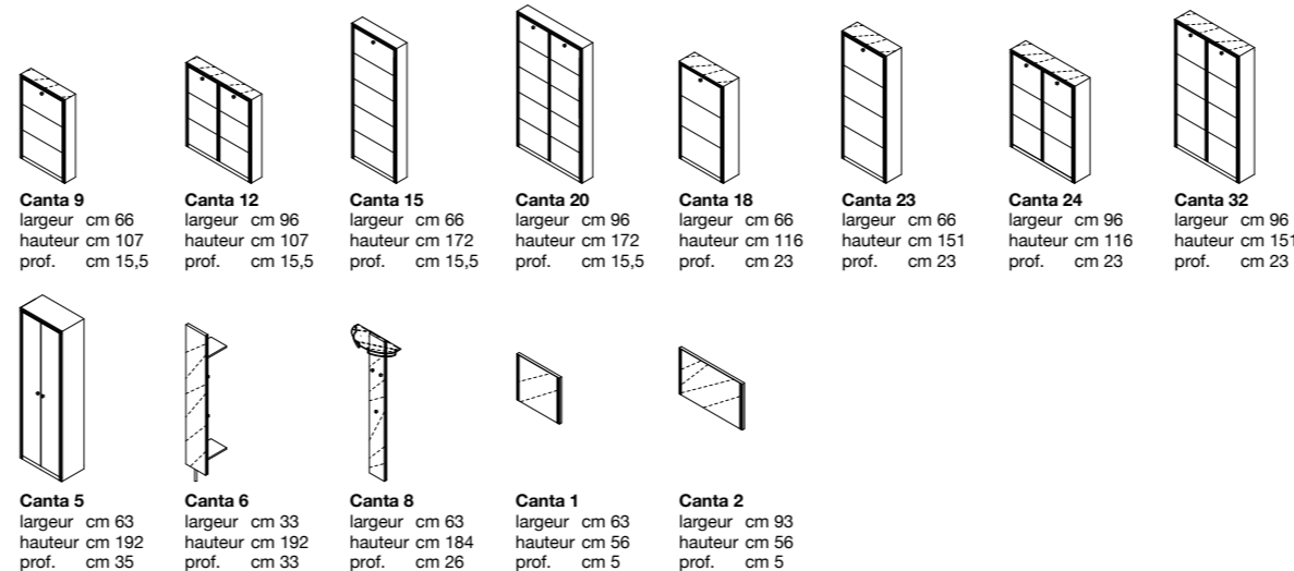
Canta 2 | Miroir (Cadre: aluminium brossé) Canta 24 | Armoire à chaussures, battants avec panier pour chaussures (Structure: aluminium mélaminée – Cadre: aluminium brossé – Fronteau: blanc lux – Top: verre blanc)
